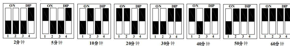
BRT-413 延时时间拨码调节示意
