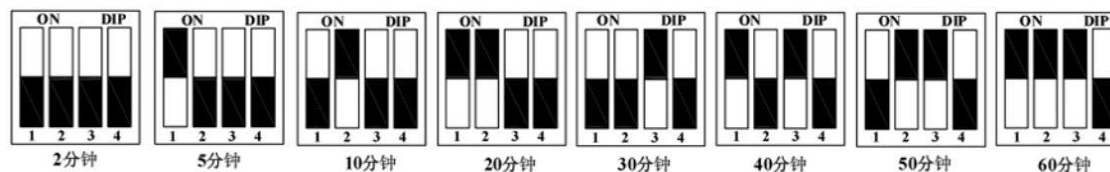
BRT-414 延时时间拨码调节示意
